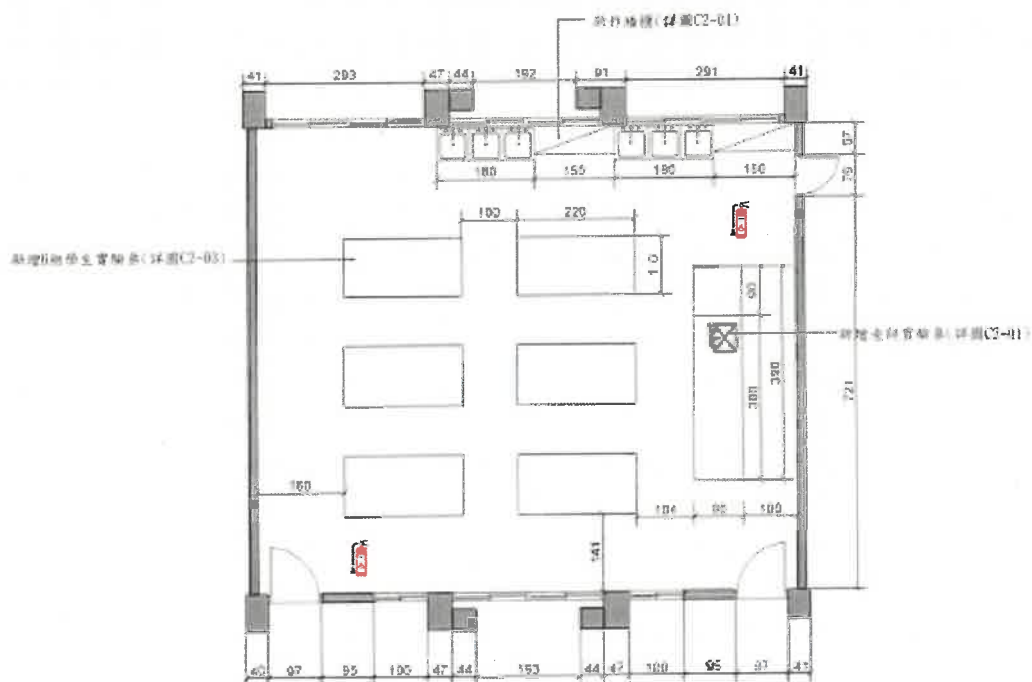
平面圖
