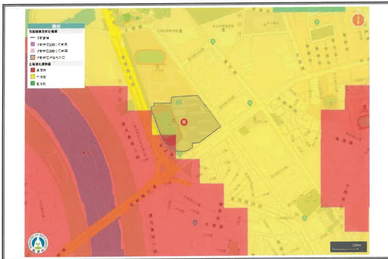
圖 2.4.1 地震災害潛勢圖 (瀏覽日期：113 年 10 月 4 日)
