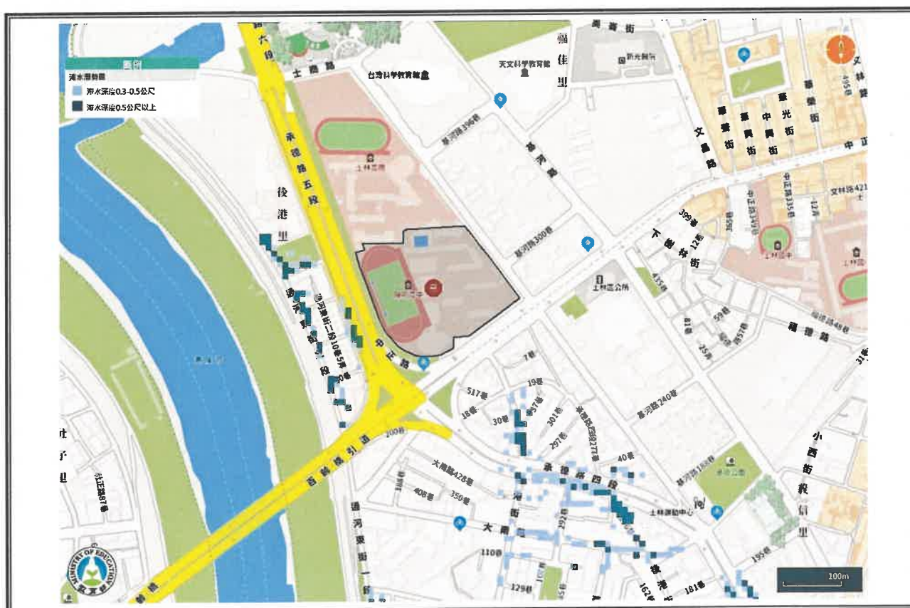
圖 2.4.2 淹水災害潛勢圖 (瀏覽日期：113 年 10 月 4 日)
